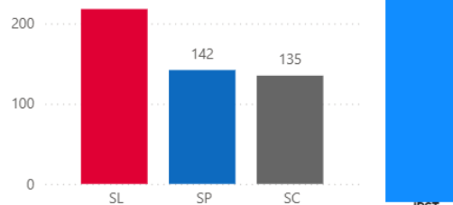
Nº de Dadores Previstos por CST
